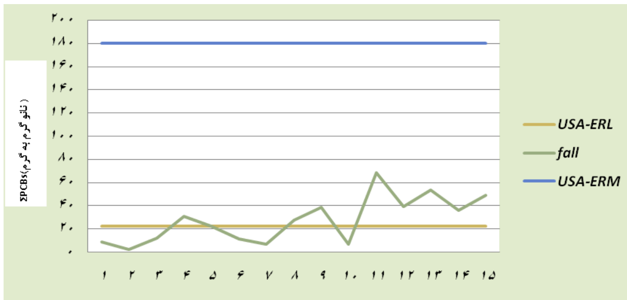
شکل ۶- نمودار مقایسه مقادیر \Sigma PCBs در رسوبات منطقه تالاب انزلی، سال ۱۳۸۸ با مقدار استاندارد محیط زیست امریکا
